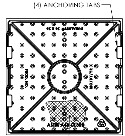
SQUARE GRID TYP ON BOTTOM
