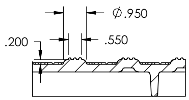
SECTION D-D SCALE 1 : 4
